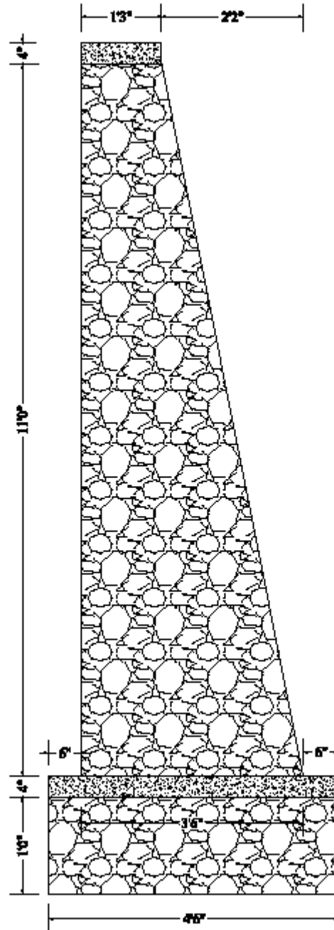
SECTION (SCALE-1"=8')
